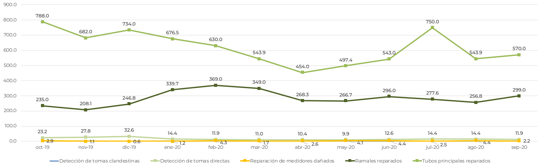
VOLUMEN RECUPERADO POR TIPO DE ACCIÓN REALIZADAS PARA DISMINUIR LA PÉRDIDA DE AGUA (LITROS POR SEGUNDO DE AGUA RECUPERADA) octubre 2019 - septiembre 2020
